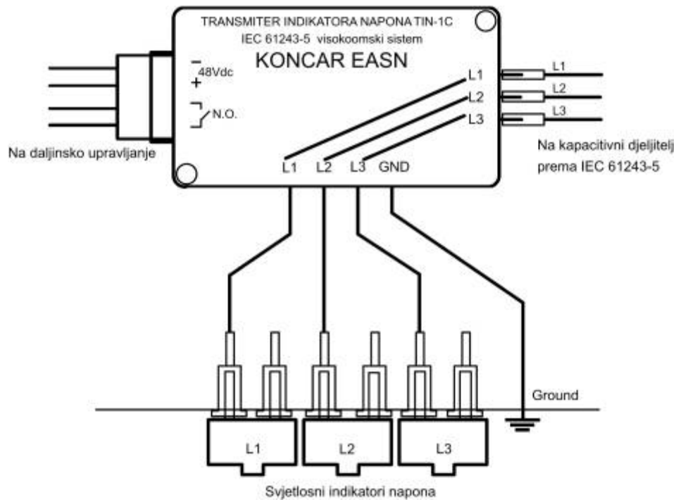
Shema spajanja
